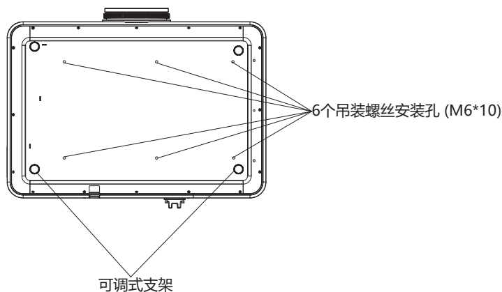
吊装螺丝安装孔及可调节式支脚的位置
